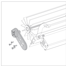
❷ ใช้ประแจหกเหลี่ยม ถอดฝา ด้านซ้ายออก
